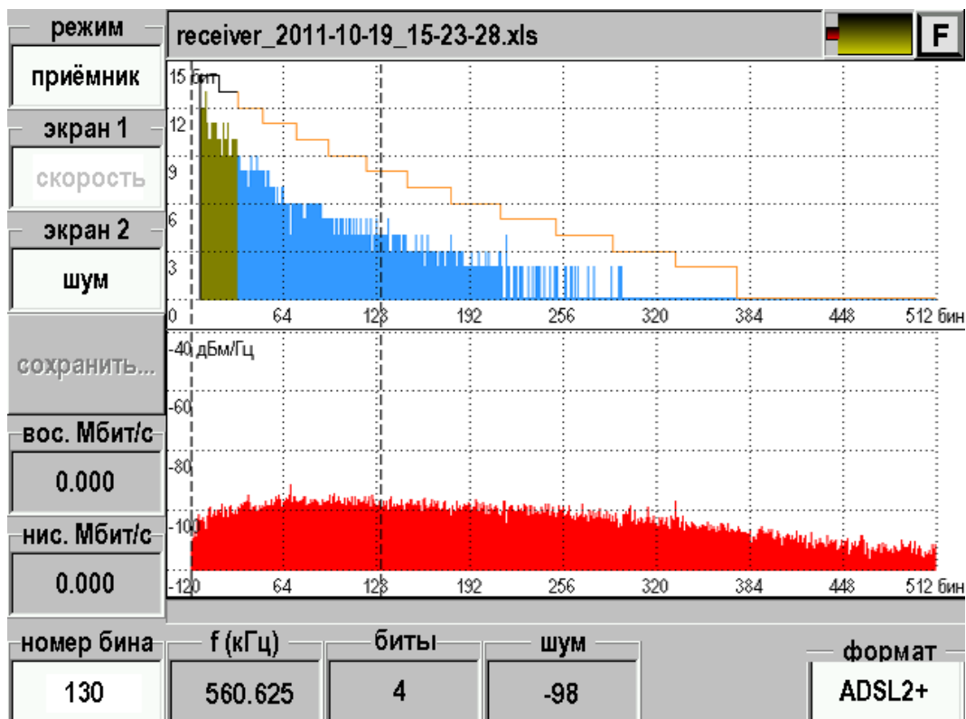
Рис. 29. Приемник. ADSL2.
