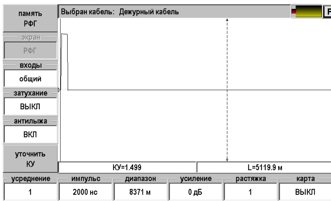
Рис. 9. Экран рефлектометра.
